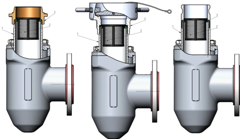
Рис.2 1- патрубок устройства слива 2-БРС (VK-80, "КАМЛОК тип А", MC-80(ПНСК), MC-2Н «ПОРШЕНЬ») 3-фильтрующий элемент с прокладкой
